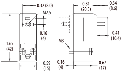
DIN Connector 43650 Form C
